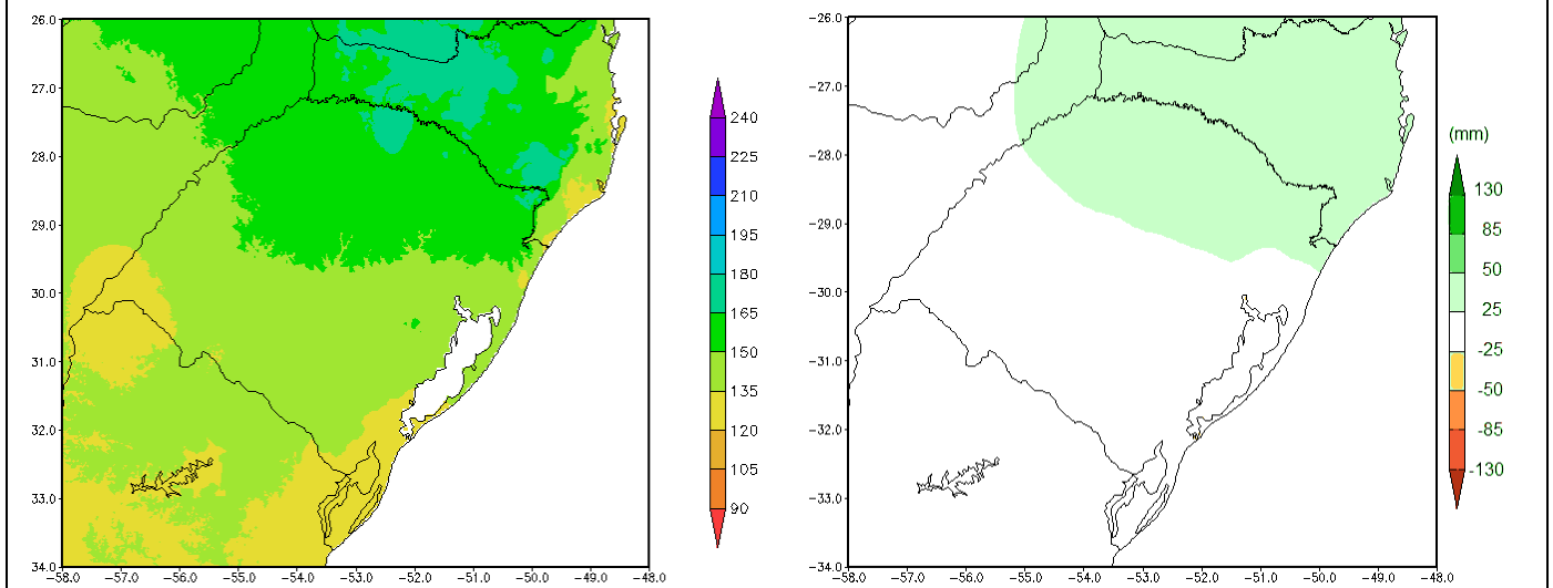
Figura 5. Chuva Média Climatologia e Anomalia Prevista junho/2019
