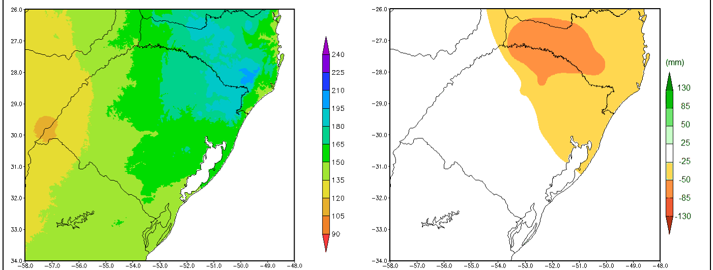
Figura 6. Chuva Média Climatologia e Anomalia Prevista julho/2019
