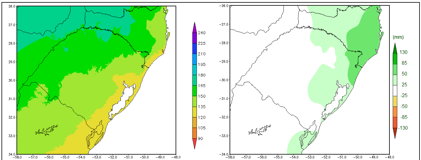
Figura 4. Chuva Média Climatologia e Anomalia Prevista maio/2019
